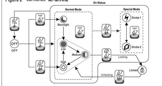
Figure 2 User interface 用户操作界面
